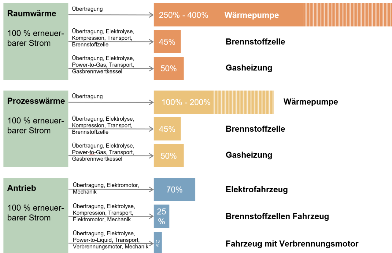
Abbildung 2: Gesamtwirkungsgrade für Raumwärme (orange, Prozesswärme (gelb) und Antriebe in der Mobilität (blau) ausgehend von erneuerbarem Strom. Gepunktete Darstellung bei der Prozesswärme weist auf die Bandbreite hin, die sich je nach Temperaturniveau ergibt. Quelle: technischer Grundlagenbericht
