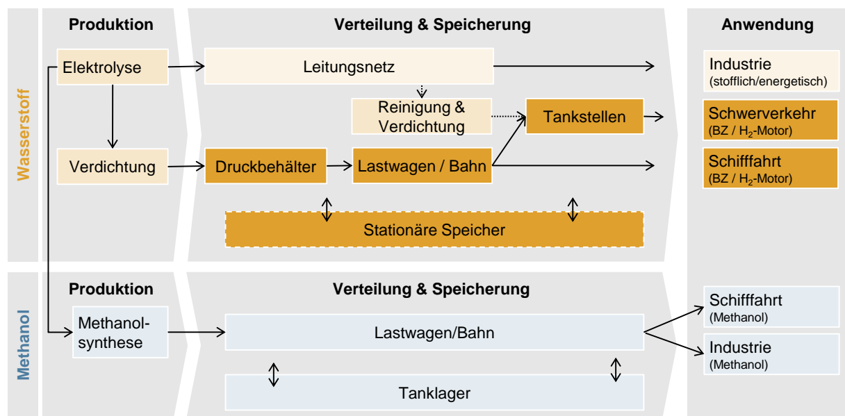
Abbildung 3: Elemente einer Infrastruktur für Wasserstoff (oben) und Methanol (unten) für die Industrie, den Schwerkverkehr und die Schifffahrt (BZ = Brennstoffzelle), ohne die Nutzung für die Stromproduktion (z.B. Methanol in Reservekraftwerken). Obere Hälfte der Abbildung: Je dunkler der Farbton, desto höher die typische Druckstufe der Anwendung. Quelle: technischer Grundlagenbericht
