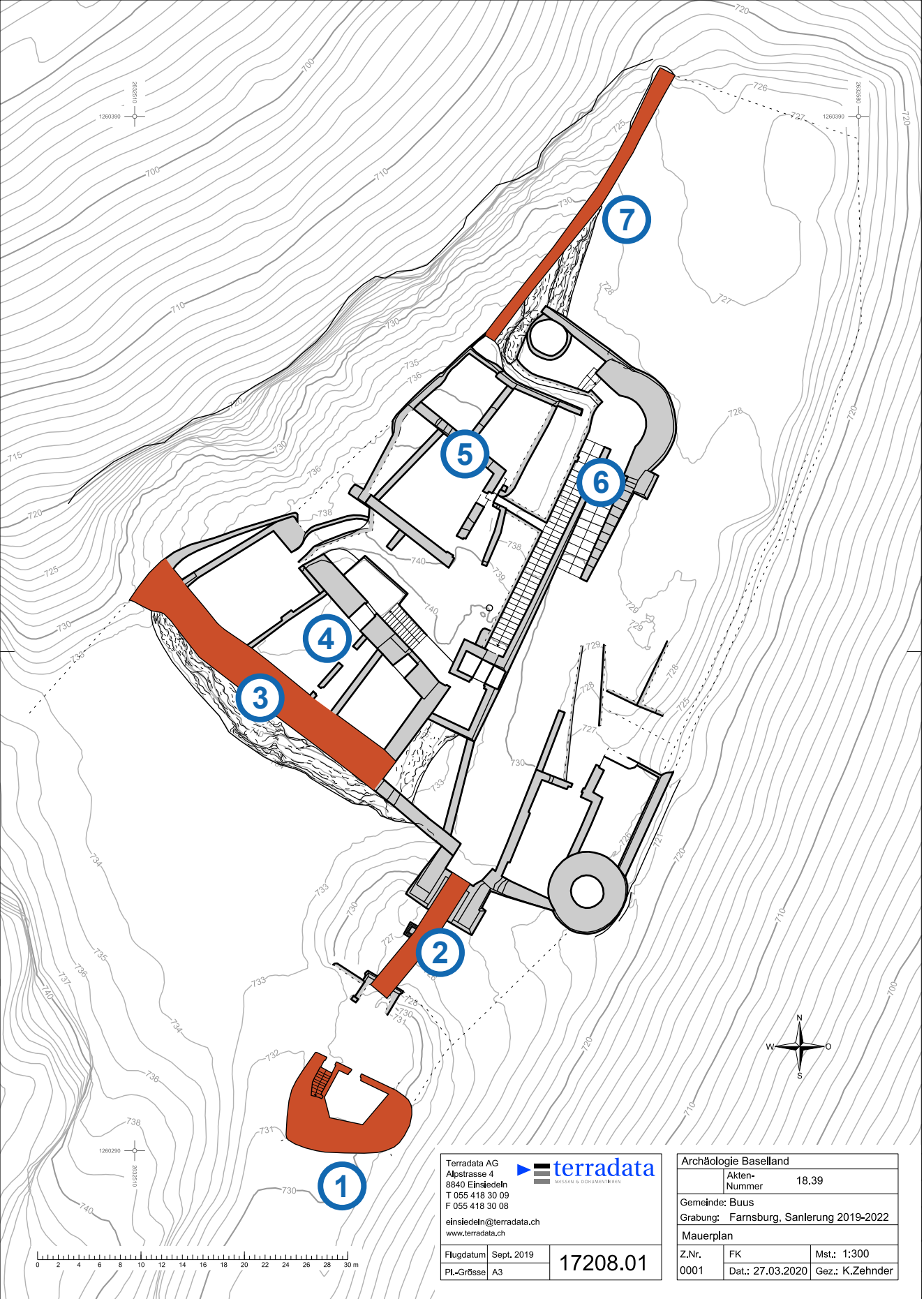
Farnsburg, Lokalisierung der im Text erwähnten Bauteile 1 Vorwerk (Barbakane), 2 Brücke über den Burggraben, 3 Schildmauer, 4 Palas, 5 Amtshaus, 6 Blauer Turm und Lange Stiege, 7 Ringmauer der Unterburg
